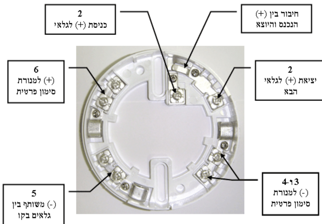
איור 1 בסיס גלאי תוצרת usVtech
