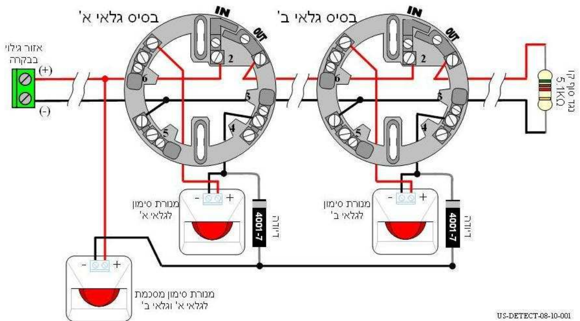
איור 5 חיבור נורת סימון מסכמת
