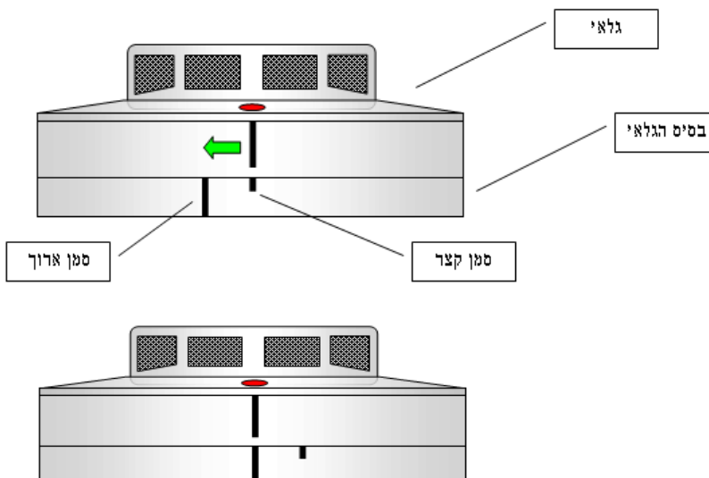
איור 2 חיבור גלאי usVtech לבסיס
