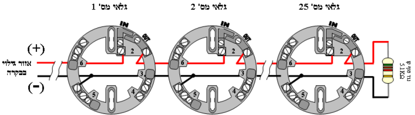
איור 3 חיבור גלאים באזור גילוי
