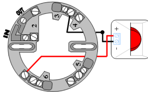
איור 4 חיבור נורת סימון לגלאי
