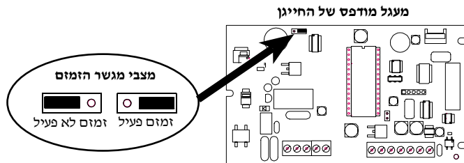
איור 2.2 - העברת מגשר הזמזום למצב "פעיל" / "לא פעיל"
